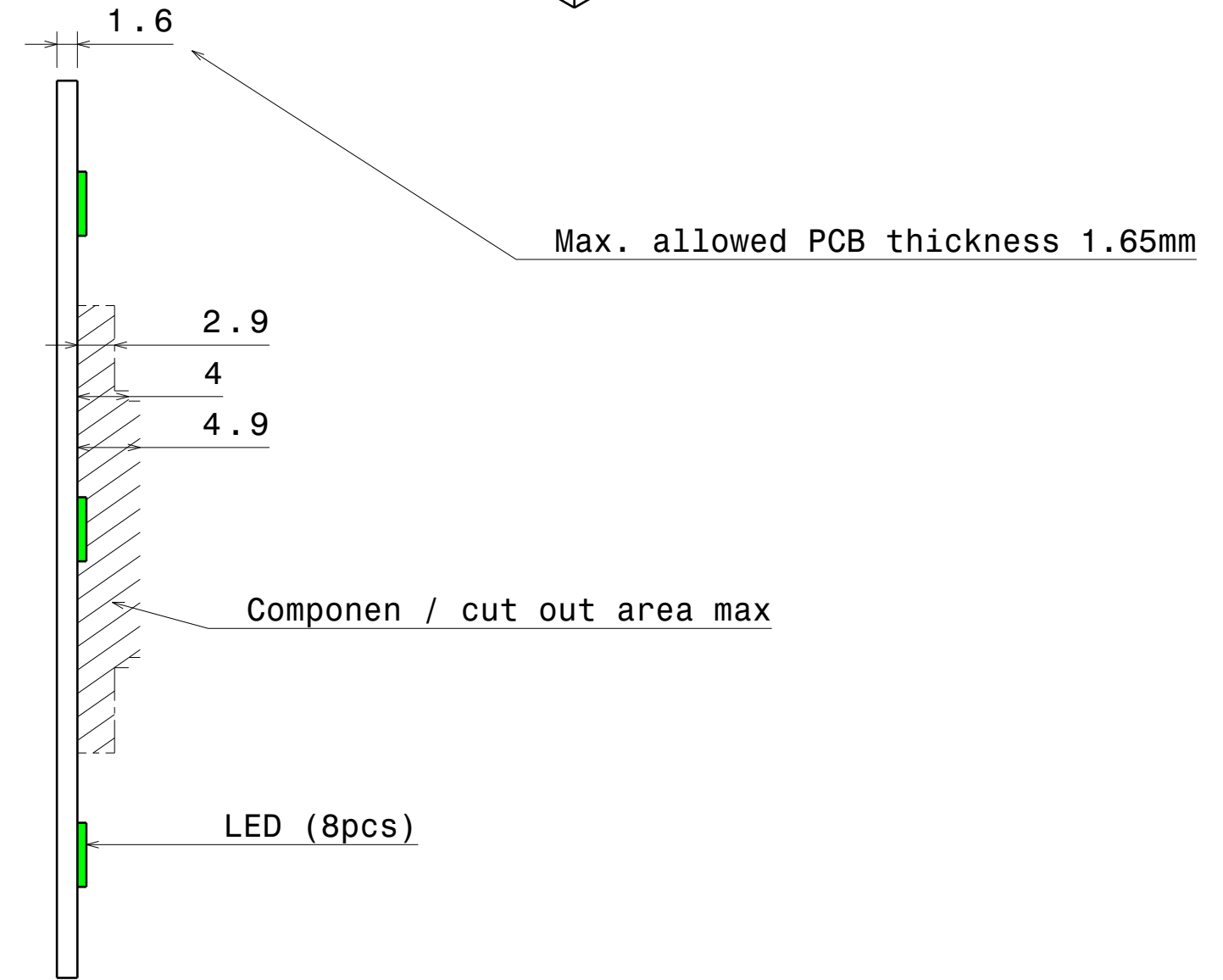
Left view Scale: 2:1
